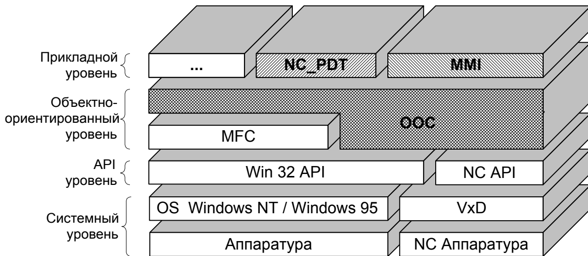
Рис. 3. Виртуальная модель PC подсистемы
