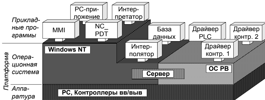
Рис. 2. Открытая архитектура систем типа PCNC
