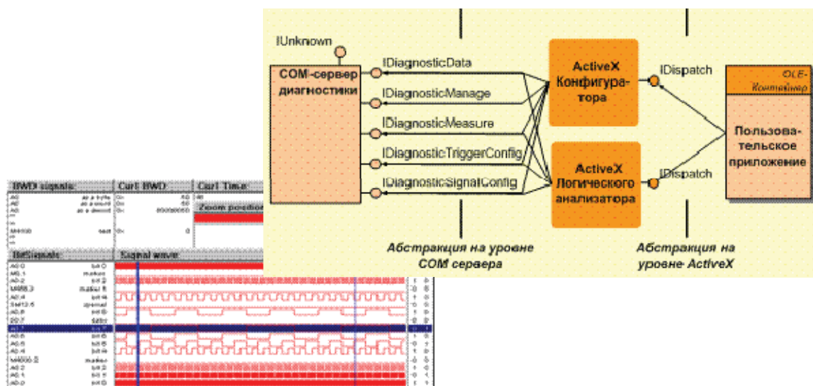
Рис.2. Логический анализатор
