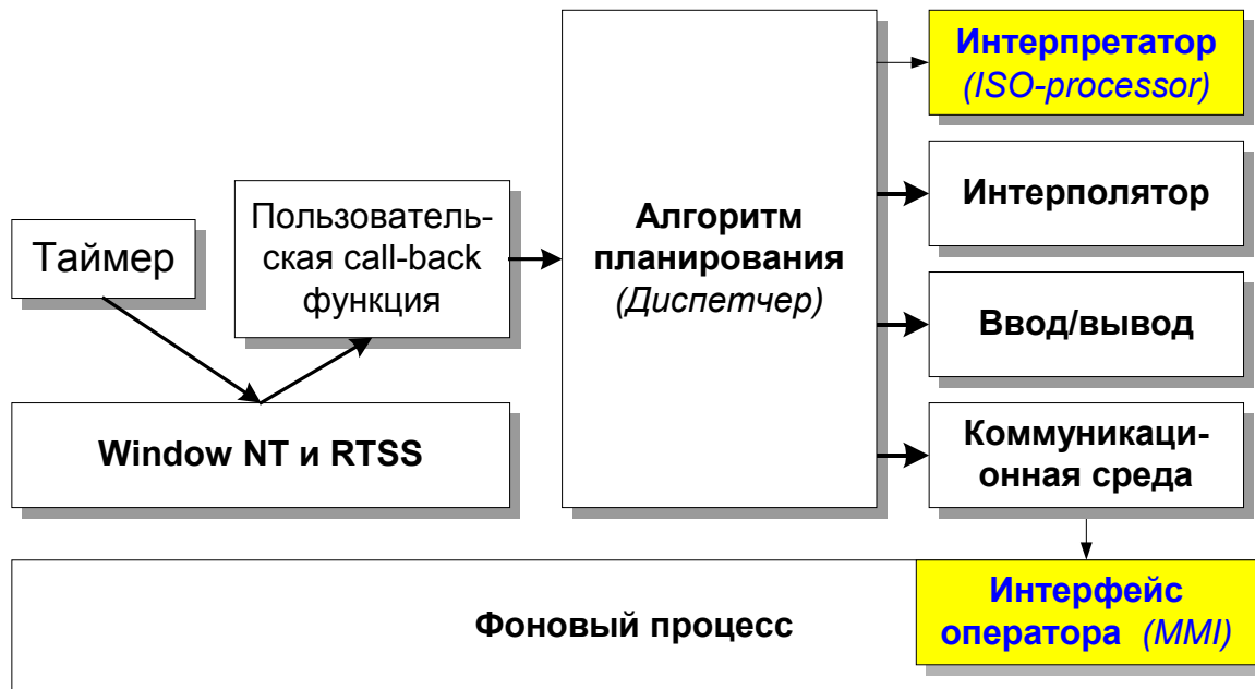
Рис. 2 Стратегия диспетчеризации задач реального времени PCNC-системы
