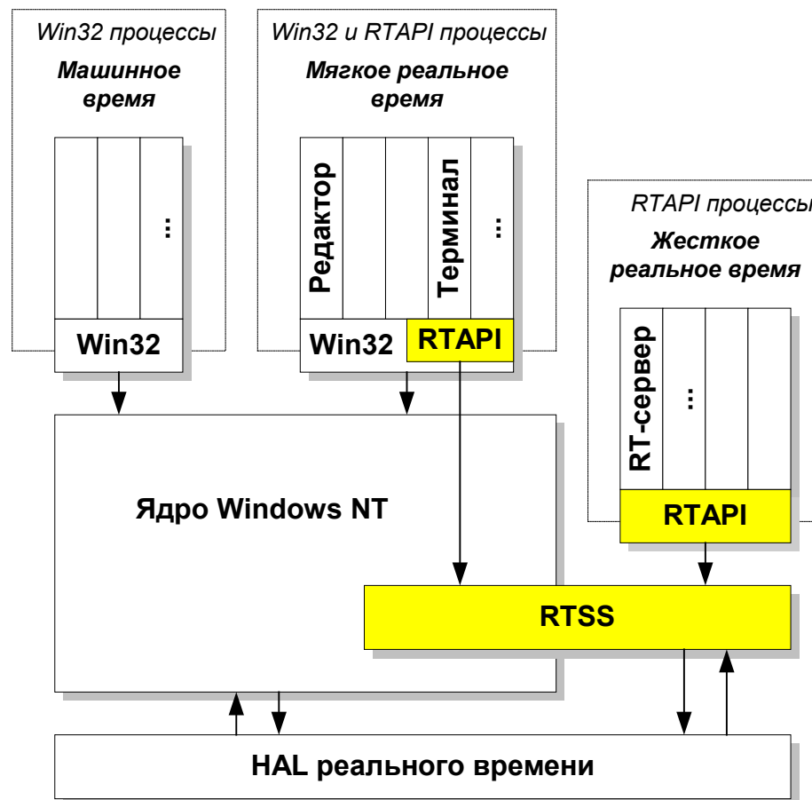
Рис. 1 Основные потоки PCNC системы в структуре Windows NT с RTX
