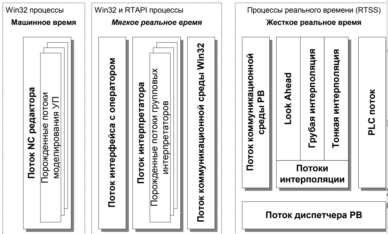
Рис. 3. Потоки PCNC системы
