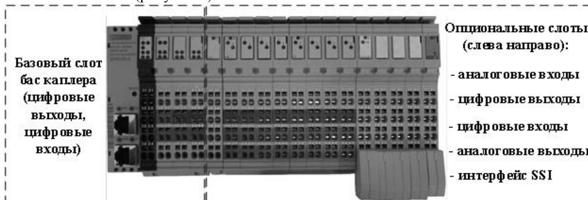
Рисунок 1 – Модуль удалённого ввода/вывода на примере бас-каплера производства компании Phoenix Contact
