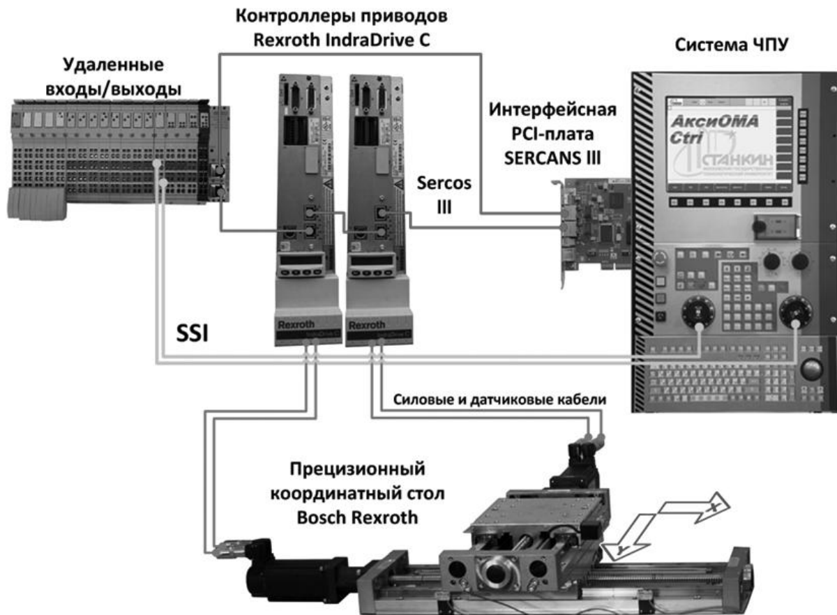
Рисунок 4 – Пример использования модуля удаленного ввода-вывода
